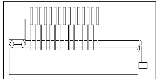
Figura 14. Montaje experimental empleado para las pruebas
