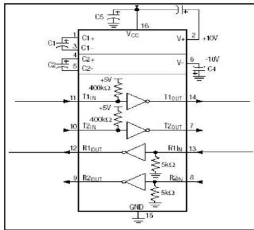
Figura 4. Diagrama eléctrico interno y conexiones del MAX232
